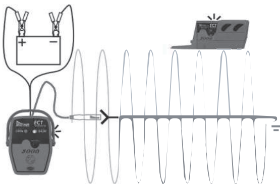
Komplettes Stromkreissignal
